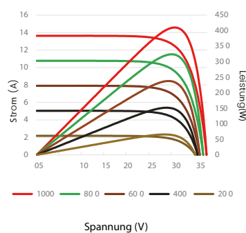
Strom-Spannungs- und Leistungs-Spannungs-Diagramme(435W)
